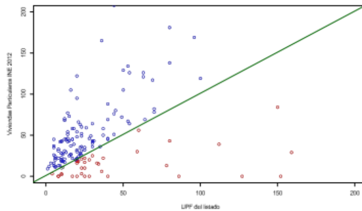
Figura 1: Scatter de las UPF del listado versus las viviendas particulares del INE 2012
